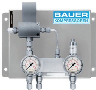
Zuschaltautomatik
